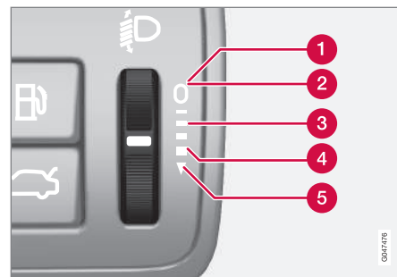
Θέσεις περιστροφικού ρυθμιστή για διαφορετικές περιπτώσεις φορτίου.
