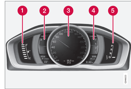
Δείκτες και ενδεικτικές λυχνίες, θέμα Elegance.
