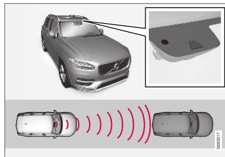
Localização da unidade de câmara e de radar 69 .
