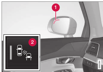
Localização das lâmpadas BLIS 75 .
