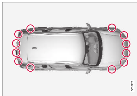
Localização dos sensores de estacionamento 128 .
