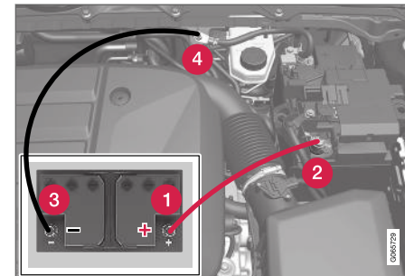
Pontos de fixação dos cabos de arranque.
