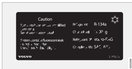
❸ 使用 R134a 冷媒車輛的空調系統資訊。
