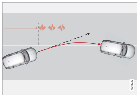
車道維持輔助功能會利用方向盤震動 111 來發出警告。
