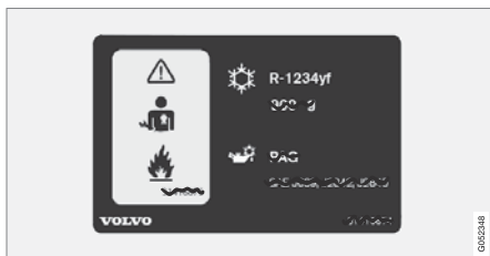
❷ 使用 R1234yf 冷媒車輛的空調系統資訊。
