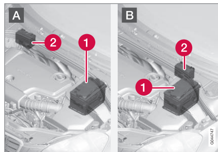
A: Automóvil con volante a la izquierda. B: Automóvil con volante a la derecha. (1). Batería de arranque 16 (2). Batería de apoyo.
