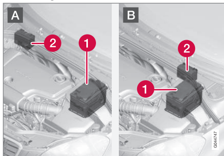
A: Modelos com volante à esquerda. B: Modelos com volante à direita. (1) Bateria de arranque 16 (2) Bateria de apoio.
