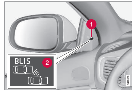
Colocación de la lámpara BLIS 38 .
