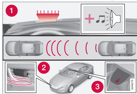
1. Zvuková a světelná výstražná signalizace v případě rizika kolize. 25
