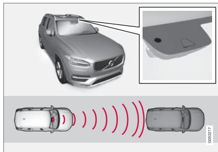
攝影機與雷達單元測量與前車的距離。
