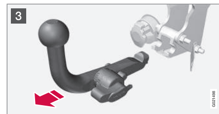
3 Fordítsa le teljesen a zárókereteket, amíg az meg nem akad. Tartsa ebben a helyzetben, miközben hátra- és felfelé húzza a vonóhorogot.
