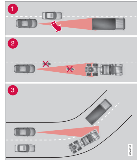
Πεδίο ορατότητας ACC.
