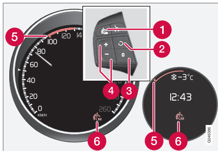
Clavier au volant et combiné d'instruments numérique ou analogique.
