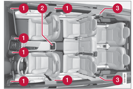
乘客室內的可調式空氣通風孔位置。
