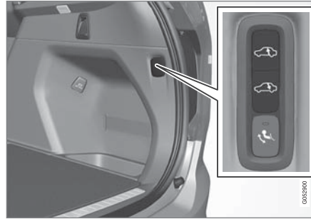
車身後段降低/升高的控制裝置
