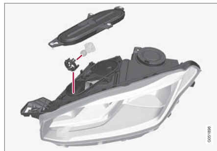
右頭燈。
