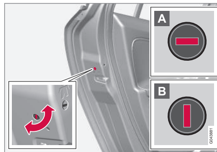
Verrouillage manuel d'une porte. À ne pas confondre avec le Verrouillage de sécurité enfant (p. 194).
