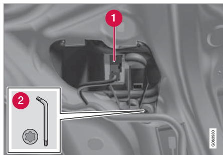
בית הפנס בצד ימין עם מכסה.
