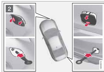
Dépose des caches avant et arrière
