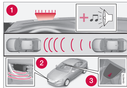
1. Lampka i dźwięk ostrzegawczy układu ostrzegającego o ryzyku kolizji 6 .
