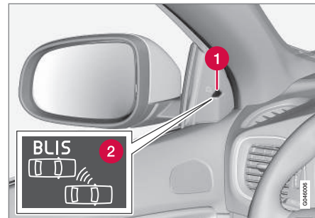
Localização da lâmpada BLIS 32 .
