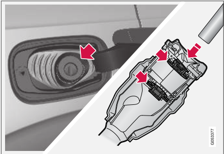
주유를 시작하기 전에 펌프 노즐을 주입구의 2개의 개방식 해치를 지나도록 배치하는 것이 중요합니다.
