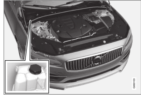
냉각수 탱크, 좌측 운전 차량.
