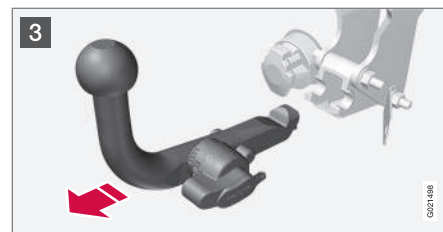
3 Повністю поверніть блокувальне колесо вниз до упору. Утримуйте його в цьому положенні, при цьому потягніть буксирувальний брус назад і вгору.
