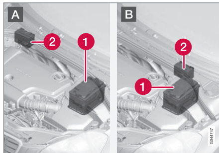
А: Лівостороннє кермо. В: Правостороннє кермо. (1) Акумулятор стартера 14 (2) Допоміжний акумулятор.
