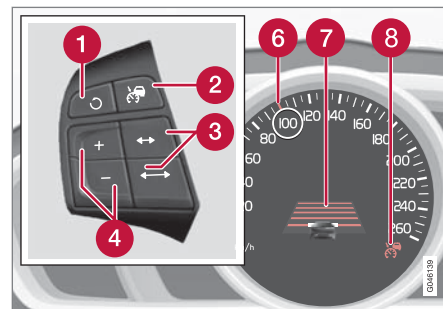
不具速度限制器的主動式定速巡航控制 9 。
