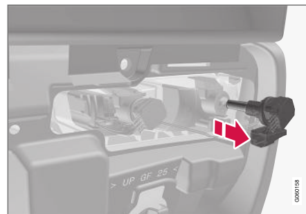
Vasemmanpuoleinen valokotelo.
