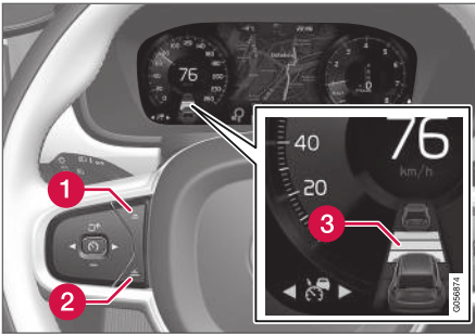
Aikaetäisyyden säädin 53 .
