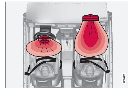
Systém airbagu při pohledu seshora, vůz s levostanným řízením.
