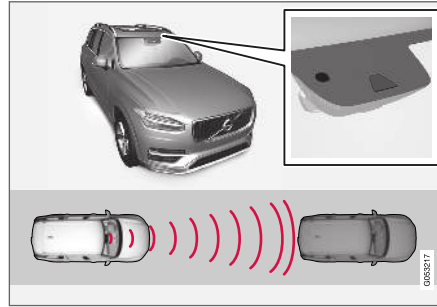
Radar ünitesinin konumu 82 .
