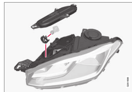
Venstre lygte.
