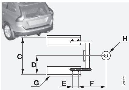
Wymiary pomiędzy punktami mocowania (mm)
