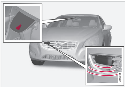
Камера та радіолокаційний датчик 25 .
