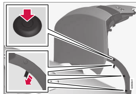
Пластмассовая защита петли крепится с помощью одной пластмассовой заклепки и трех защелок.
