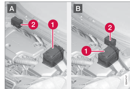
A: 左ハンドル車。B: 右ハンドル車。1. メインバッテリー 16 2. 補助バッテリー。
