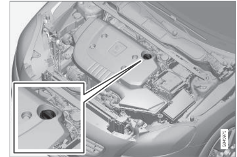
Påfyllingsrør 7 .
