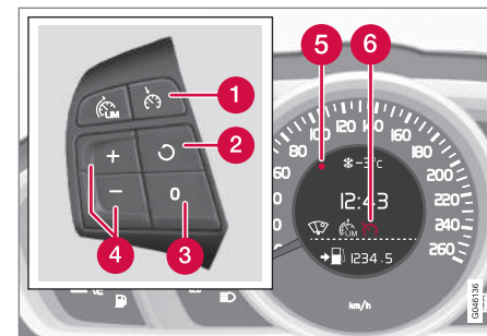
Knappene på rattet og displayet i bil med fartsbegrensere 6 .
