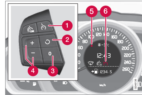
Teclado de volante y pantalla en vehículo con limitador de velocidad 9 .
