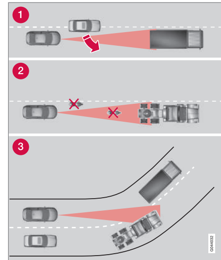
Campo de visión del ACC.
