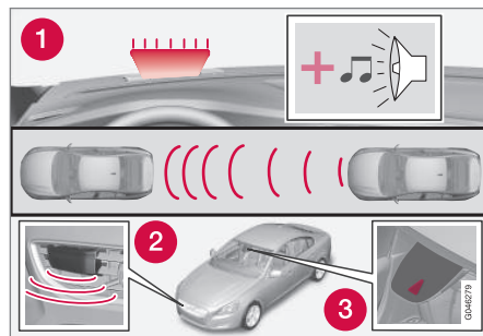
1. Señal acústica y visual cuando hay riesgo de colisión. 25
