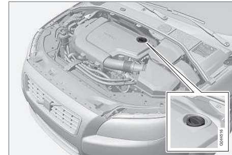
Tubo di rifornimento 7 .
