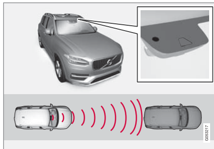
レーダーユニットの位置 81
