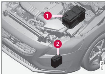
(1) Startaccu 14 (2) Hulpaccu
