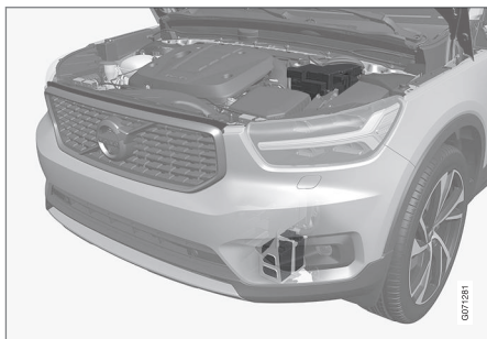
12 V stödbatteriet är placerat nere i motorrummet. Här visas också startbatteriet (överst).
