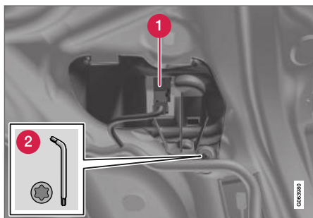
Gruppo luci con copertura sul lato destro.
