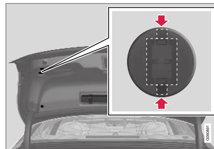
La parte rettangolare dei fermagli è orientata nel senso longitudinale dell'automobile.
