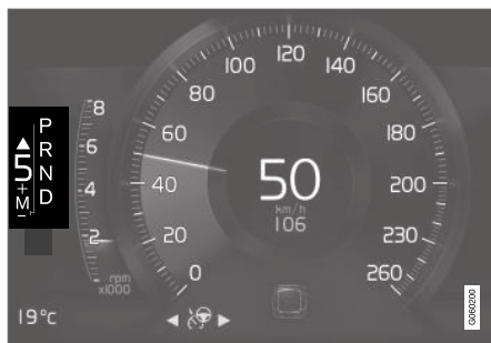
Indicatore cambio di marcia sul display del conducente da 8".
