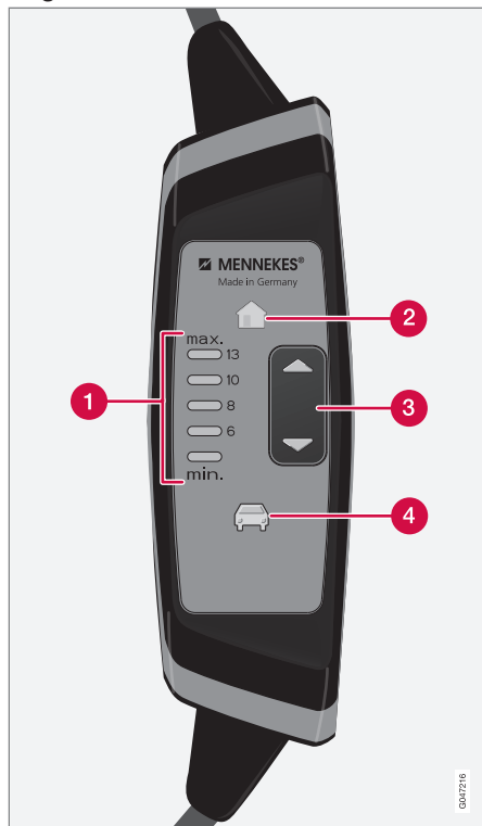
Display en bedieningstoetsen regeleenheid.
