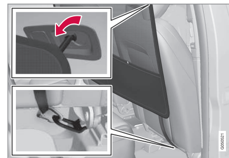
Montage voorin.
