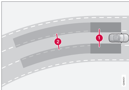
Principe voor BLIS: 1. Zone in de dode hoek. 2. Zone voor snel inhalende voertuigen.
