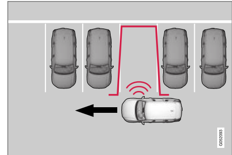
Suorakulmaisen pysäköinnin periaate.
