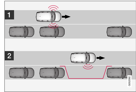
Samansuuntaisen pysäköinnin periaate.
