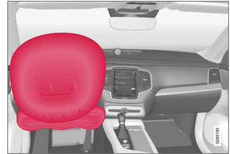
Ohjauspyörän turvatyyny ja polviturvatyyny kuljettajan istuimella.
