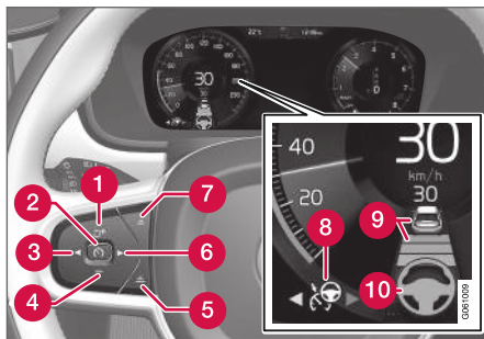
Toiminnon painikkeet ja symbolit 69 .
