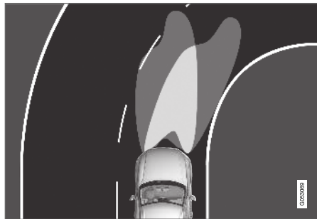
기능을 끈(좌측) 상태 및 켜(우측) 상태 각각의 전조등 패턴.
