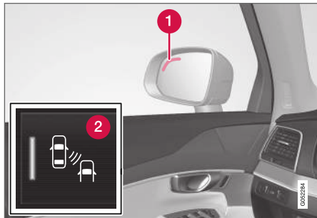
BLIS 램프 72 의 위치.
