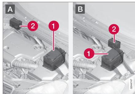
A: Samochód z kierownicą po lewej stronie. B: Samochód z kierownicą po prawej stronie. (1) Akumulator rozruchowy 14 (2) Akumulator pomocniczy.
