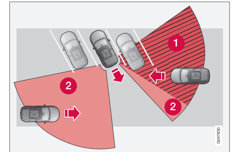
Dans les zones de stationnement à angles, le CTA peut être « aveugle » d'un côté
