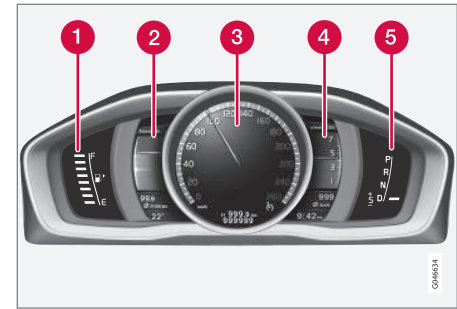
Thème Eco : jauges et témoins
