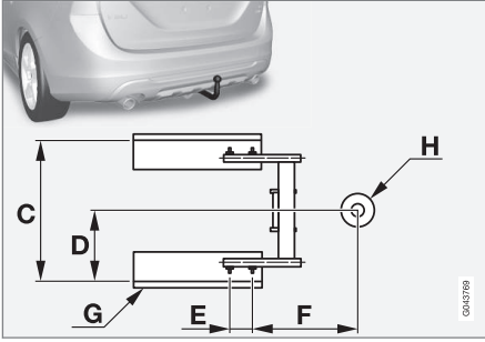
Montaj noktalarının büyüklükleri (mm)
