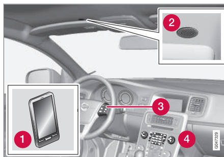
Rozmieszczenie elementów
