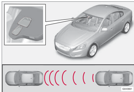
レーザーセンサーの送信/受信ウィンドウ 12
