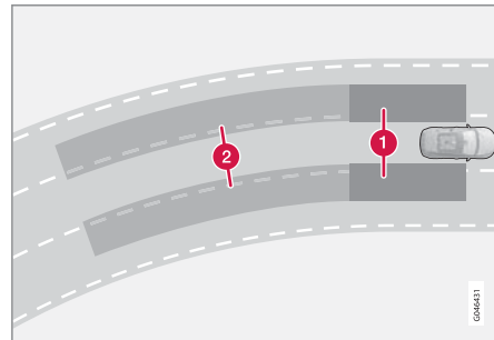
BLIS の原理：1. 死角ゾーン 2. 急接近する車両のゾーン
