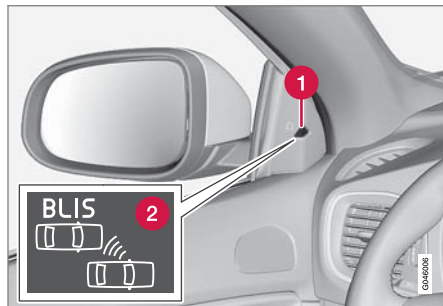
BLIS ランプの場所 22
