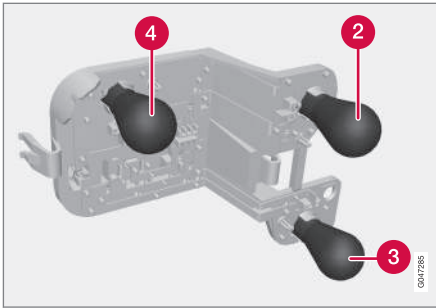
Heckleuchte, Lampenfassung
