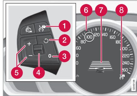
ระบบควบคุมความเร็วคงที่พร้อมการปรับความเร็วอัตโนมัติที่มีตัวจำกัดความเร็ว 9
