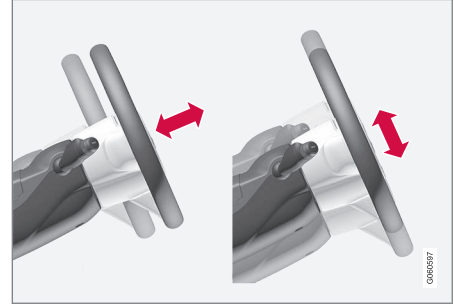
Direksiyon simidinin yüksekliği ve derinliği ayarlanabilir.
