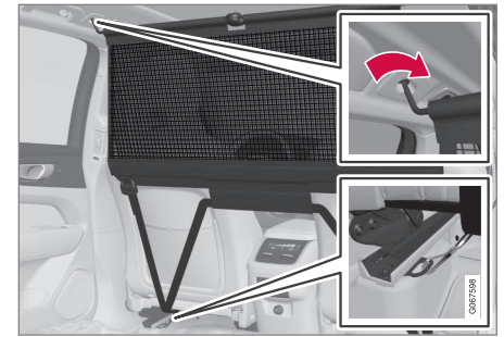
Etumainen asennus.
