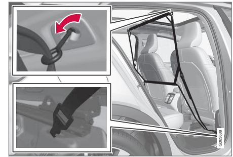
Montaje delantero.
