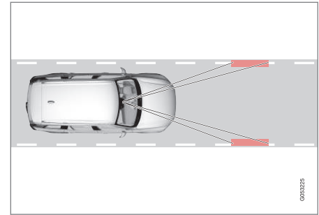
Una cámara se encarga de detectar las líneas pintadas que delimitan la vía o el carril.
